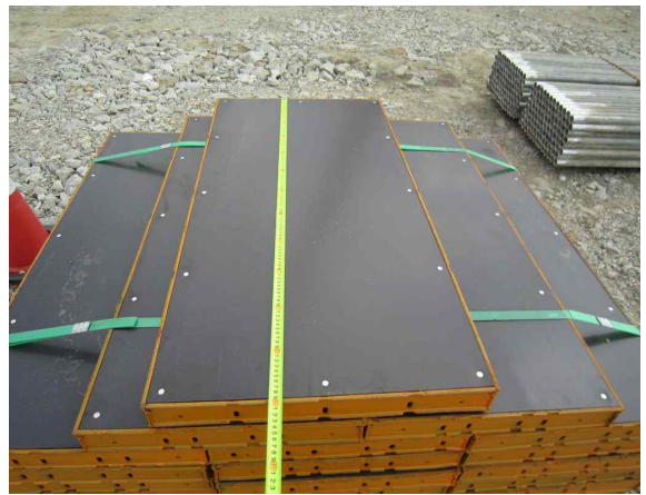
교량 A1 거푸집 자재 검수 (600×1200)
